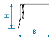
YEA endestiver. Afstiver top- og bundprofiler samt løsholter. Korrosionsklasse C2/C4.
