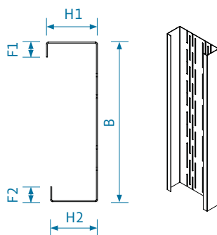
RY(K) ydervægsstolpe. Slidset stolpe placeret mellem top- og bundskinner. Korrosionsklasse C2/C4.
