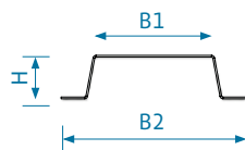
Hat-profil uden perforering. Korrosionsklasse C3 - C4.
