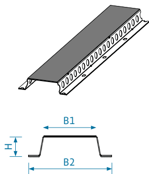
YVLP ventileret hat-profil inkl. EPDM-gummi. Afstiver top- og bundprofiler og løsholter. Korrosionsklasse C3 - C4.
